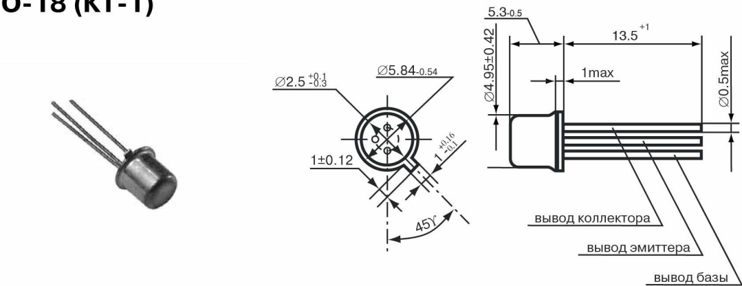
ТО-18 (КТ-1)
