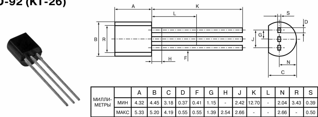
ТО-92 (КТ-26)
